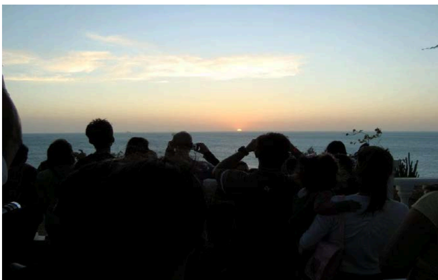
Transito de Venus GAZ-Paraguana: 05/06/2012
